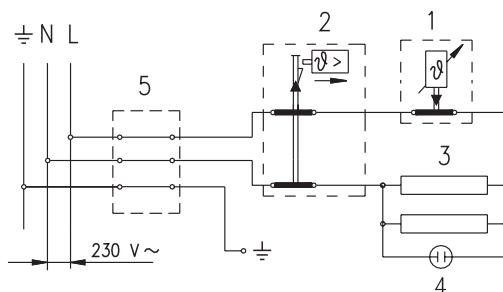
Instalația electrică
